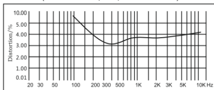
ИСКАЖЕНИЯ
