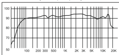
ЧАСТОТНЫЙ ДИАПАЗОН
