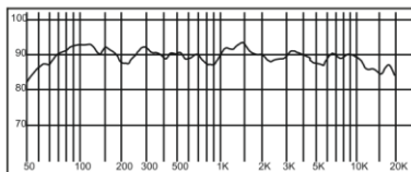
ЧАСТОТНЫЙ ДИАПАЗОН (dB SPL, 1W, 1m)
