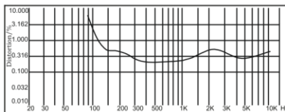
ИСКАЖЕНИЯ (THD < 1.5% 1W, 1m, 100Hz-16kHz)
