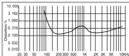
ИСКАЖЕНИЯ (THD < 1.5% 1W, 1m, 200Hz-10kHz)
