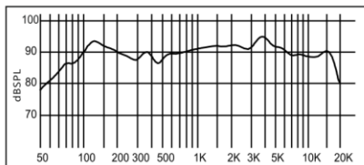
ЧАСТОТНЫЙ ДИАПАЗОН (dB SPL, 1W, 1m)
