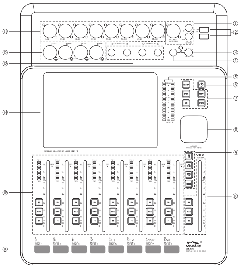
(Панель микшера DM20)
