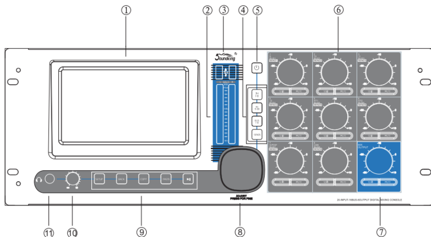
(Передняя панель микшера DB20P)
