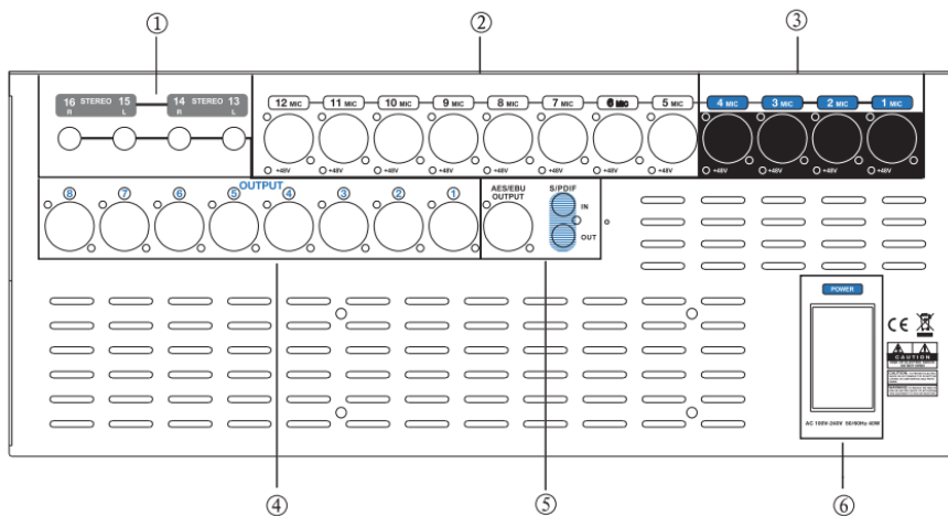
(Задняя панель микшера DB20P)
