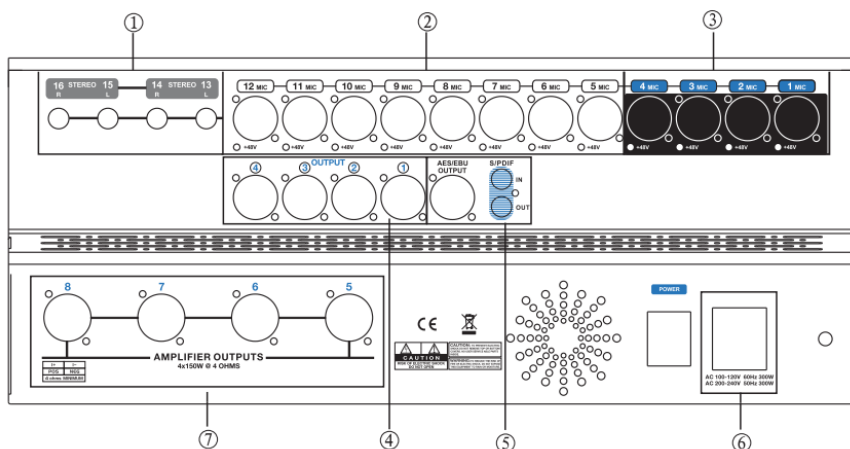
(Задняя панель микшера DB20P-600)
